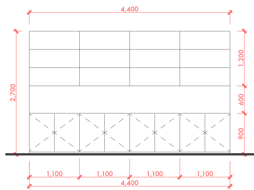
POHLED
