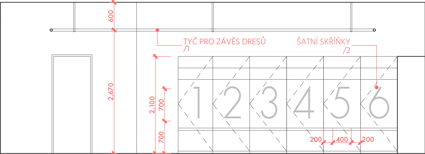
S.29/A | ŠATNA A-TÝM
