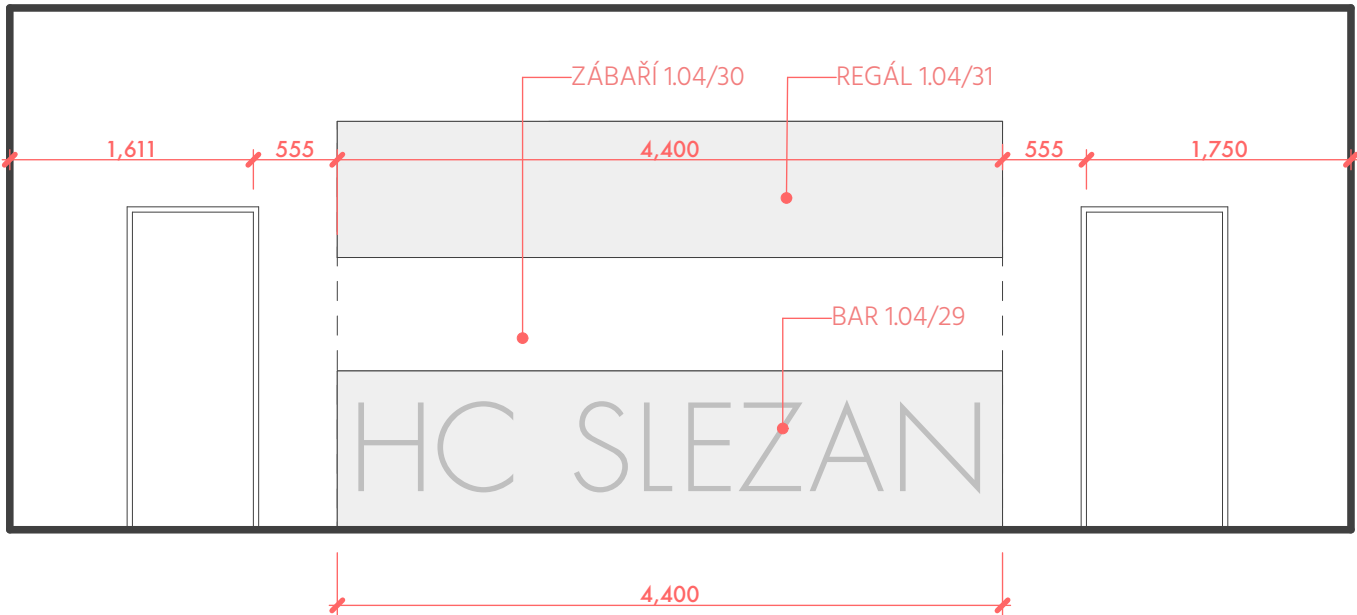
1.04/A | POHLED NA BAR
