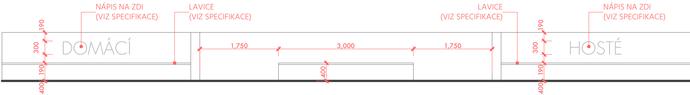
TRESTNÉ LAVICE
