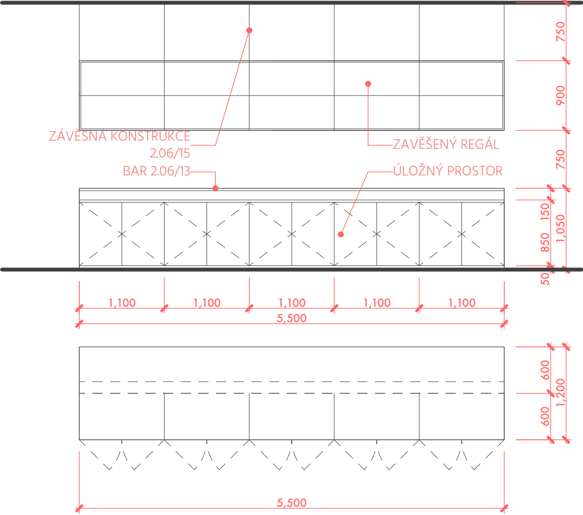
2.06/C | BAR + HORNÍ REGÁL
