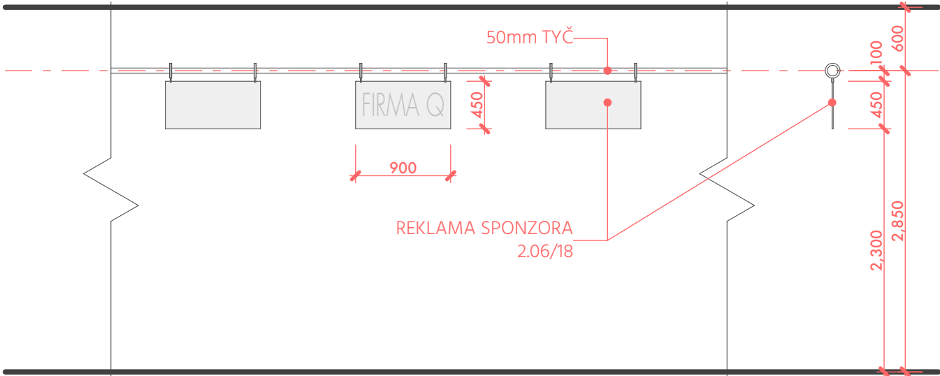
2.01/10 | PROFIL PRO ZAVĚŠENÍ REKLAMY SPONZORA
