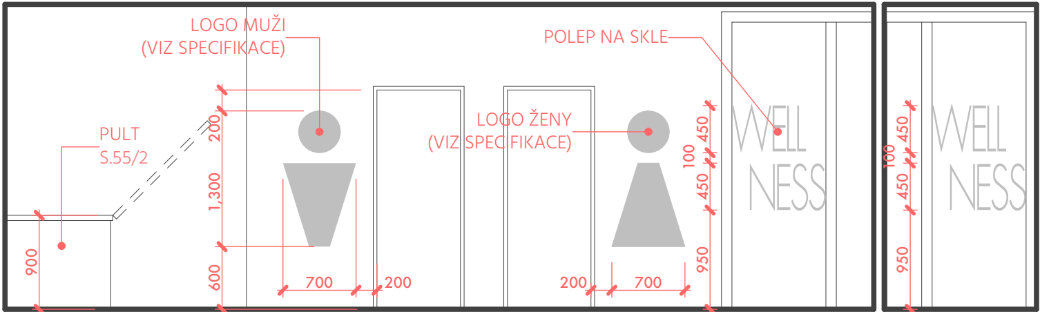
S.53/B + S.52/B | ŠATNA / CHODBA
