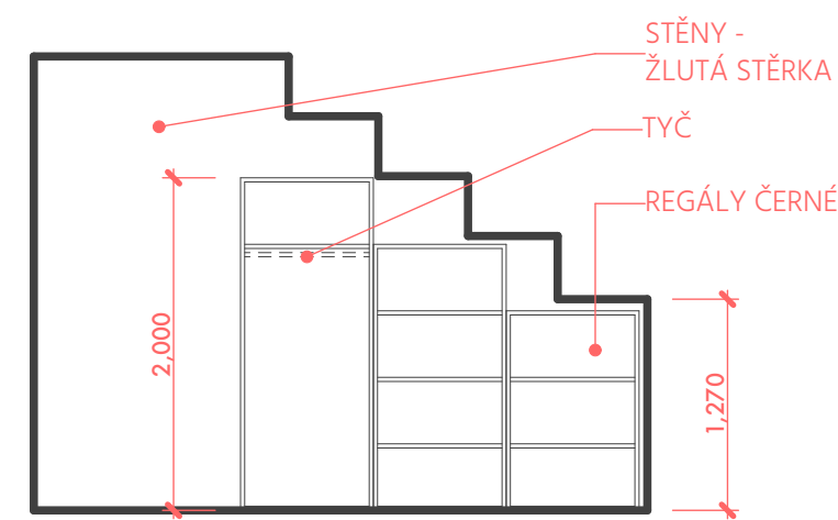
1.40/A | POHLED NA REGÁGLY 1.40/1
