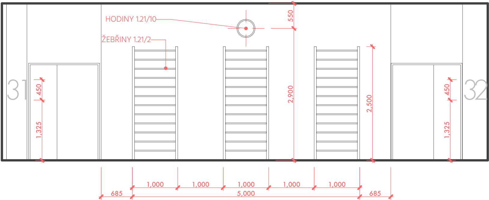
1.21/B | TĚLOCVIČNA
