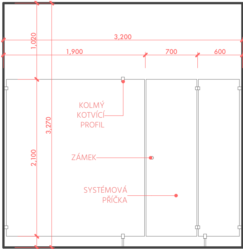
S.30/A | SKLAD
