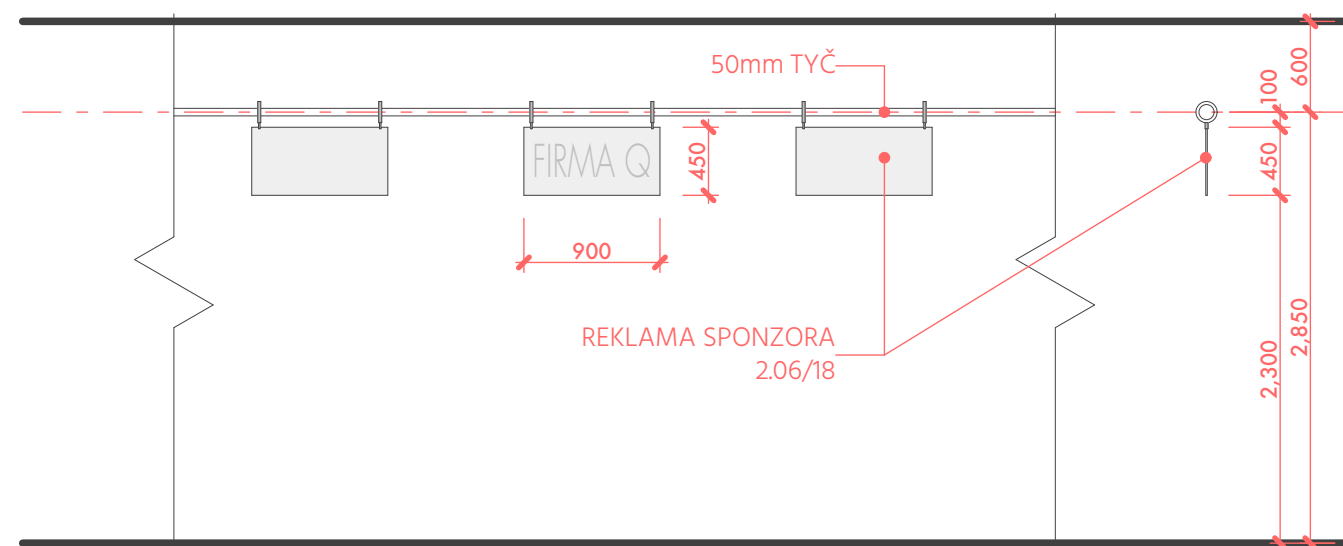
2.06/18 | PROFIL PRO ZAVĚŠENÍ REKLAMY SPONZORA
