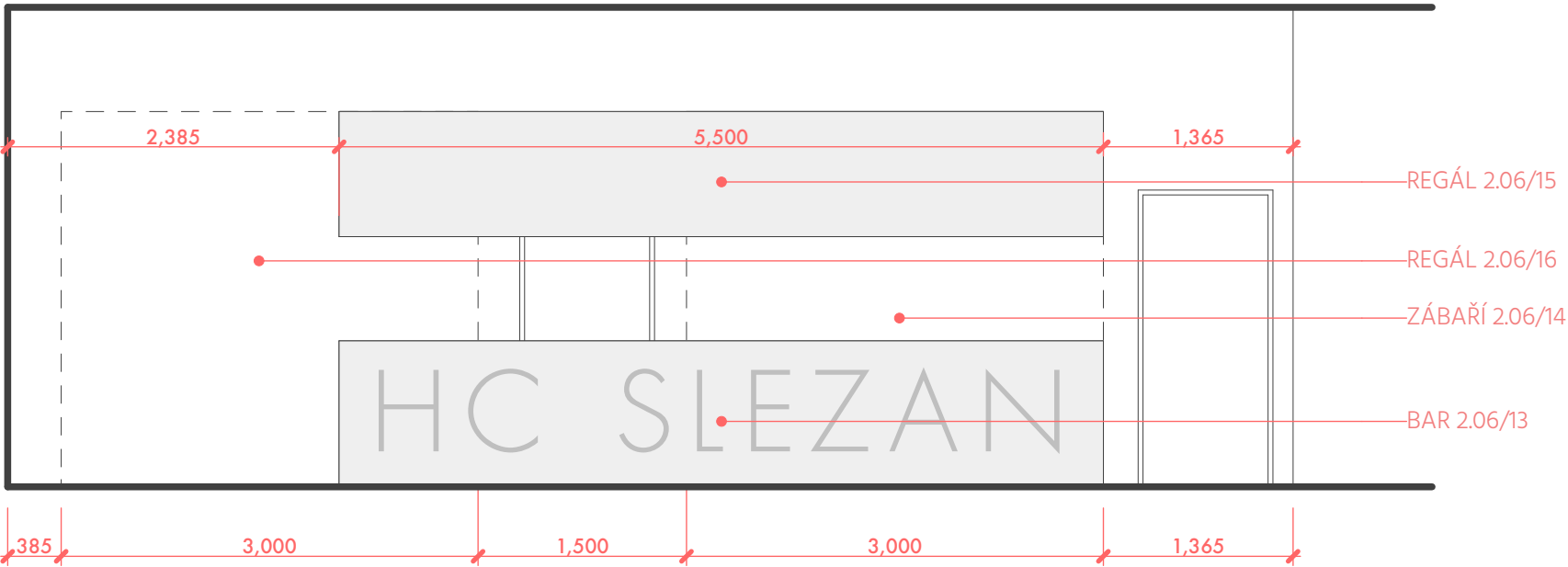
2.06/A | POHLED NA BAR
