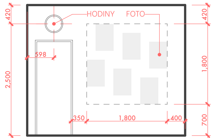
S.65/A + S.66/A | MASÉRNA
