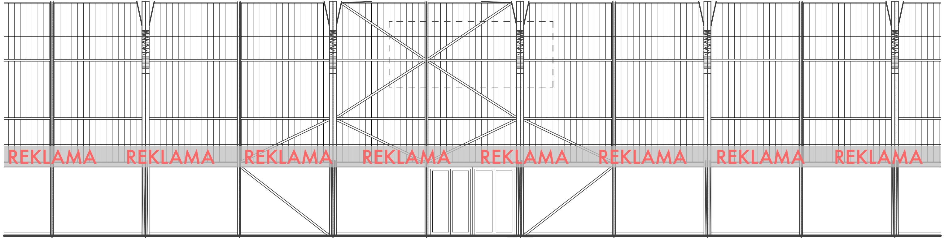
1.34/8 | REKLAMNÍ PÁS - POHLED
