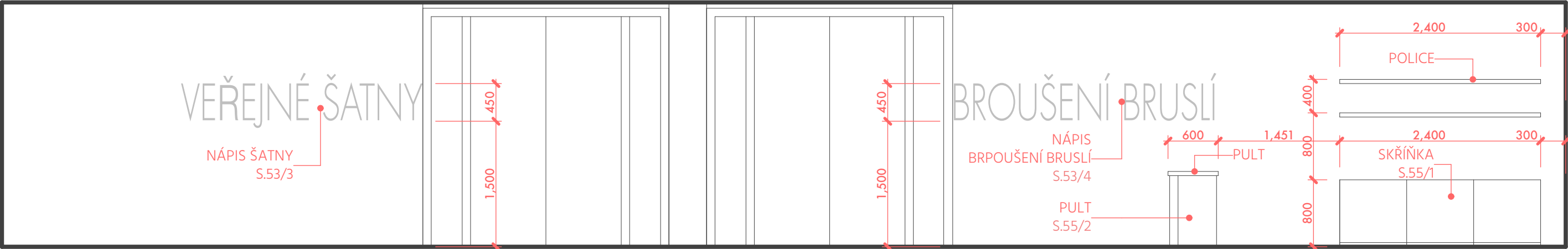
S.53/A + S.55/A | ŠATNA
