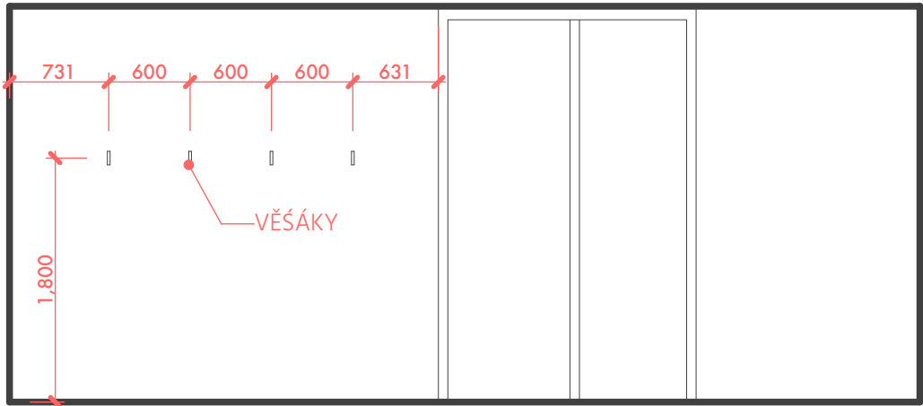
S.67/A | SPRCHY
