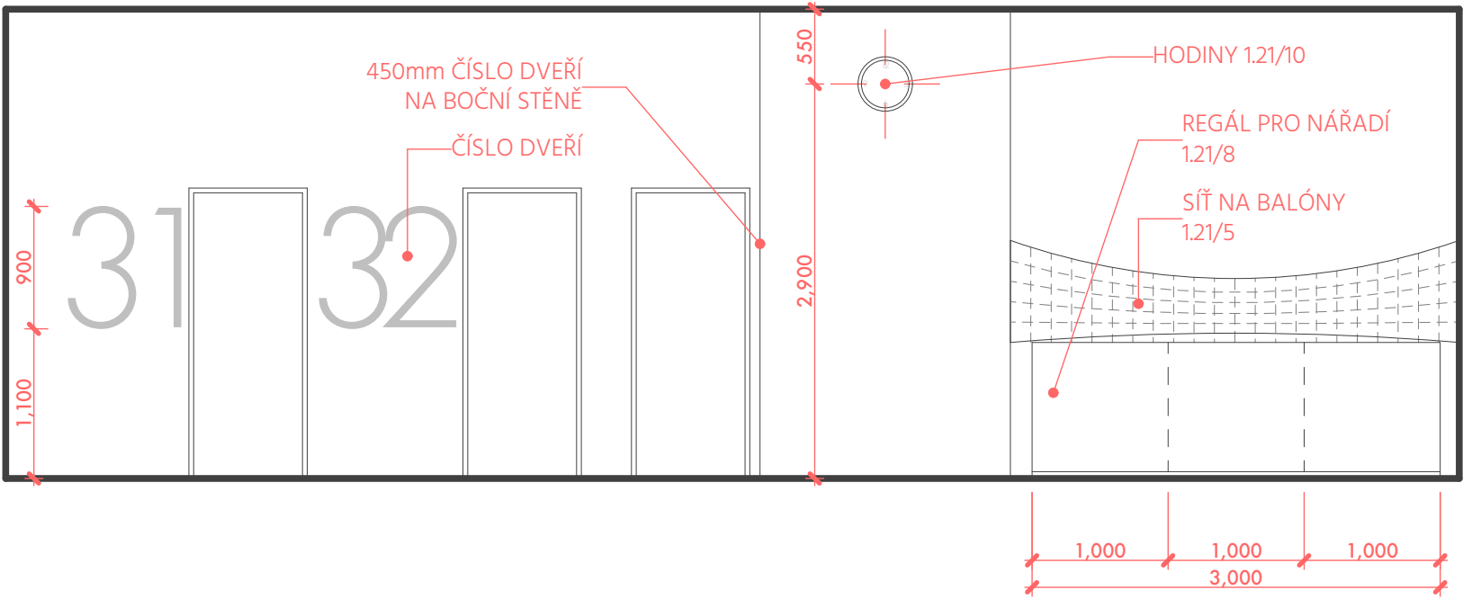
1.21/A | TĚLOCVIČNA
