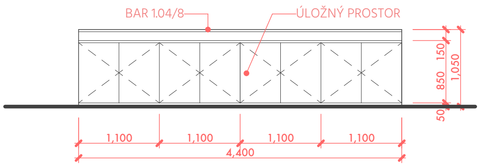
POHLED Z BARU
