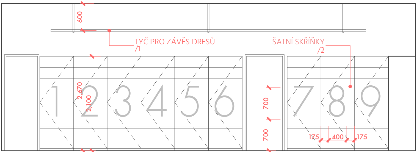
A | TYPICKÁ ŠATNA
