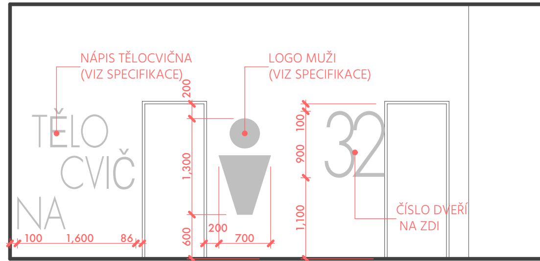
1.01/A | VSTUPNÍ HALA
