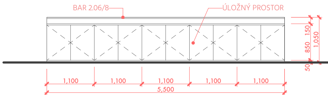
POHLED Z BARU
