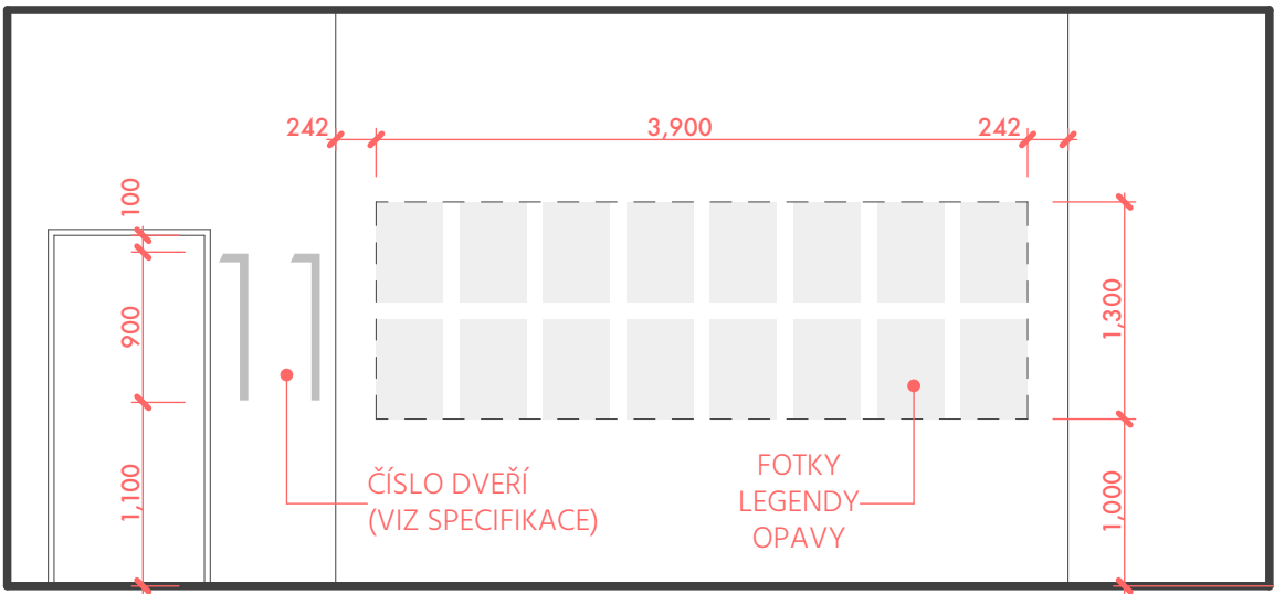
2.10/D | HALA
