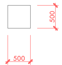
SKŘÍŇKA 1.40/3 - POHLED A PŮDORYS
