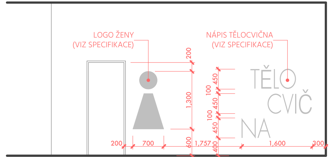
1.01/B | VSTUPNÍ HALA
