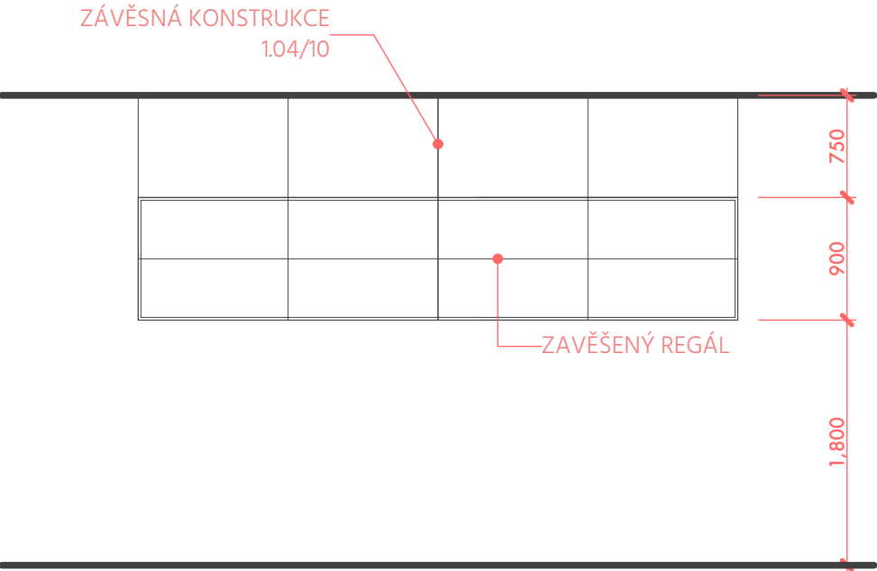
POHLED Z BARU
