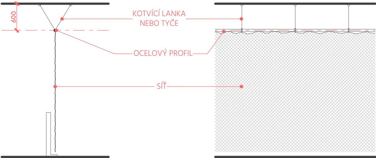
2.01/9 | SÍŤ - ŘEZ
