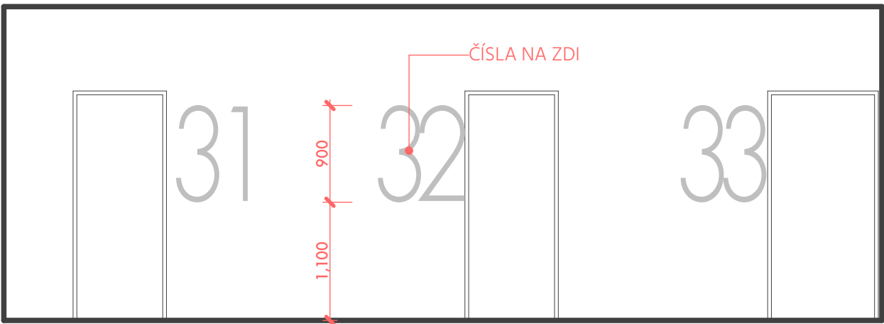
S.64/B | CHODBA
