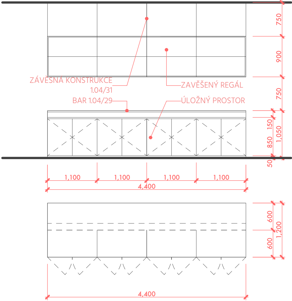
1.04/C | BAR + HORNÍ REGÁL
