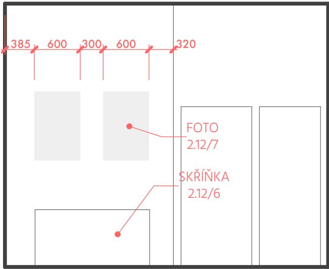
2.12/B | ZASEDACÍ MÍSTNOST
