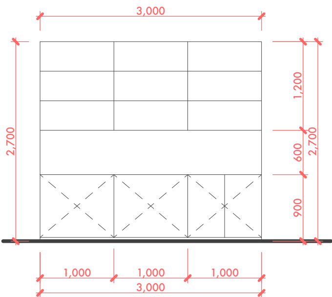
POHLED
