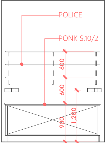
S.10 | MALÁ BRUSÍRNA - POHLED
