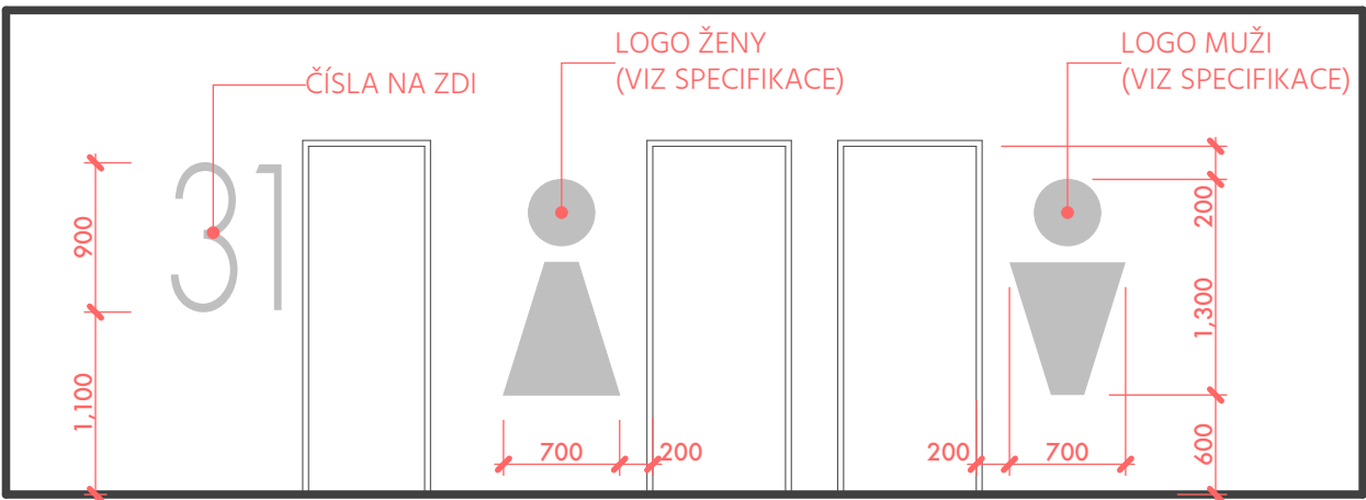
S.64/A | CHODBA
