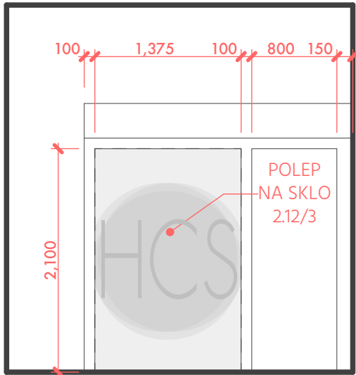
2.12/A | ZASEDACÍ MÍSTNOST
