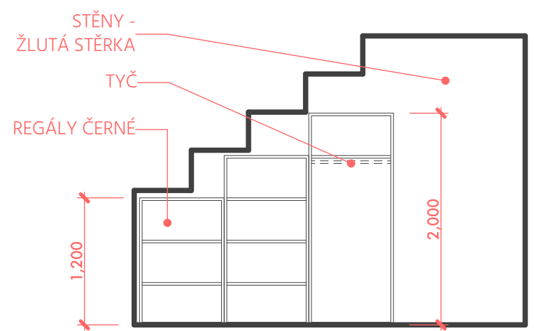
1.40/C | POHLED NA REGÁGLY 1.40/1
