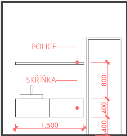
S.60/B | OŠETŘOVNA
