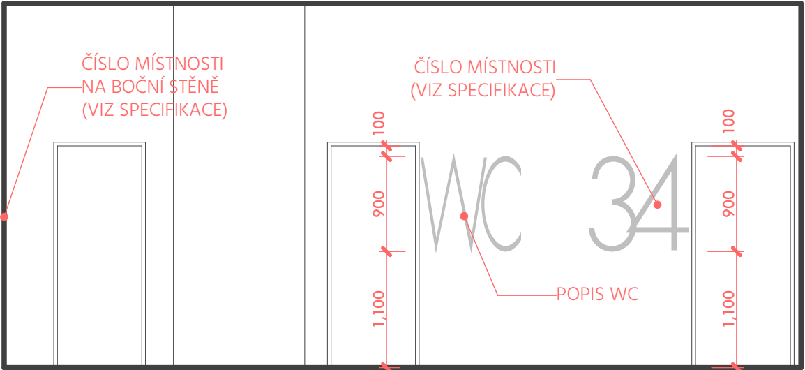
2.10/B | HALA
